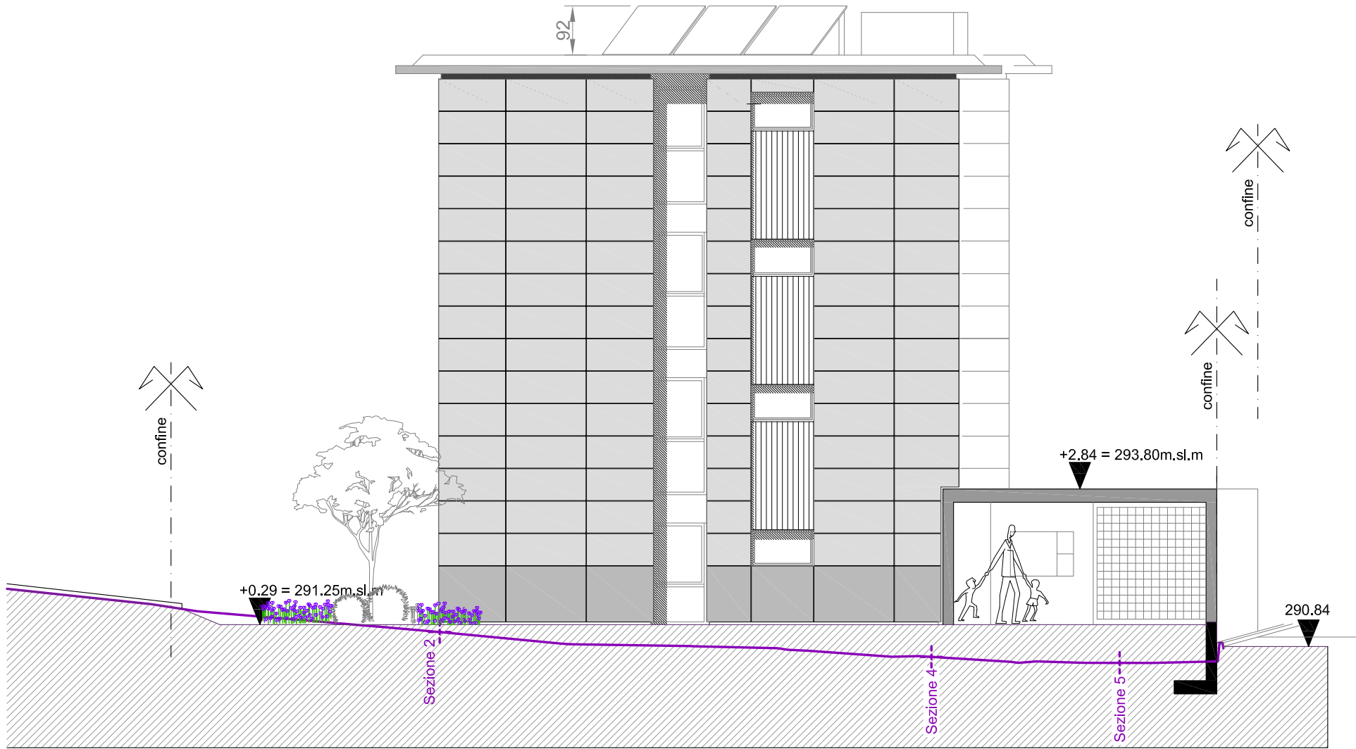
FACCIATA SUD - EST 1:100
